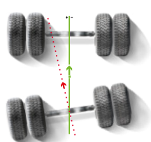
Ferdén állás
