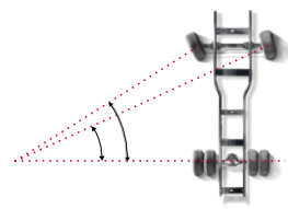
Nyomtáv szögdifferencia
